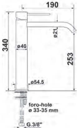
RXZ402A • MONOCOMANDO LAVABO ALTO Ø 40 MM • HIGH WASH BASIN MIXER Ø 40 MM • MITIGEUR LAVABO HAUT Ø 40 MM
