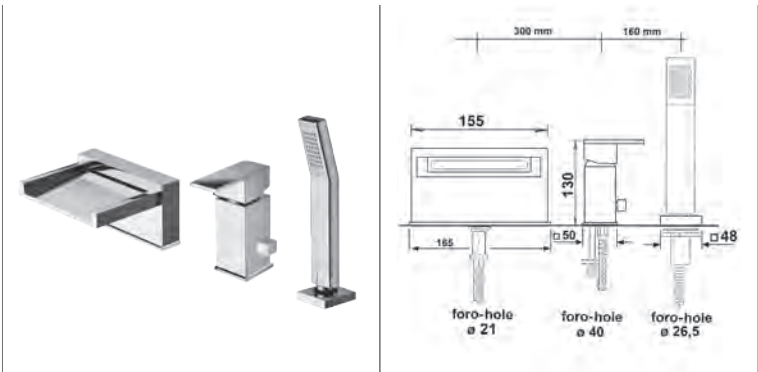
8731 • MONOCOMANDO BORDO VASCA 3 FORI CON BOCCA A CASCATA • 3 HOLES DECK MOUNTED BATH SHOWER MIXER WITH WATERFALL SPOUT • MITIGEUR BAIN-DOUCHE 3 TROUS SUR GORGE AVEC BEC CASCADE
