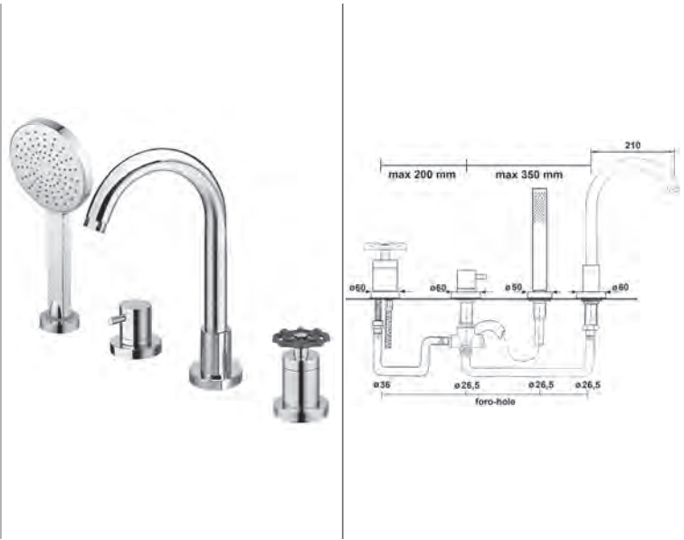
5130TT • MONOCOMANDO BORDO VASCA 4 FORI COMPLETO • 4 HOLES DECK MOUNTED BATH SHOWER MIXER WITH SHOWER KIT • MITIGEUR BAIN-DOUCHE 4 TROUS SUR GORGE AVEC ENSEMBLE DE DOUCHE
