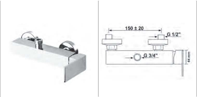
8744 • MONOCOMANDO DOCCIA ESTERNA NUDO • ONE HANDLE SHOWER MIXER WITHOUT SHOWER KIT • MITIGEUR DOUCHE EXTÉRIEUR NU
