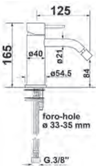
RXZ403 • MONOCOMANDO BIDET Ø 40 MM • BIDET MIXER Ø 40 MM • MITIGEUR BIDET Ø 40 MM
