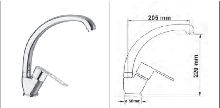
2577 Elle • MONOCOMANDO LAVELLO • ONE HANDLE SINK MIXER • MITIGEUR ÉVIER
