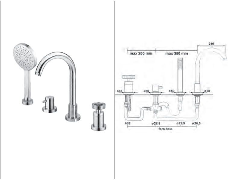
5130ZZ • MONOCOMANDO BORDO VASCA 4 FORI COMPLETO • 4 HOLES DECK MOUNTED BATH SHOWER MIXER WITH SHOWER KIT • MITIGEUR BAIN-DOUCHE 4 TROUS SUR GORGE AVEC ENSEMBLE DE DOUCHE
