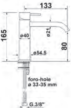
RXZ402 • MONOCOMANDO LAVABO Ø 40 MM • WASH BASIN MIXER Ø 40 MM • MITIGEUR LAVABO Ø 40 MM
