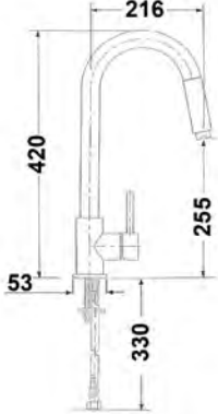
5570 Rhapsody • MONOCOMANDO LAVELLO CON DOCCIA ESTRAIBILE • MONO SINK MIXER WITH PULL-OUT HANDSPRAY • MITIGEUR ÉVIER MONOTROU AVEC DOUCHETTE EXTRACTIBLE
