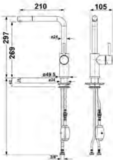
55170 Rhapsody • MONOCOMANDO LAVELLO CON DOCCIA ESTRAIBILE • MONO SINK MIXER WITH PULL-OUT HANDSPRAY • MITIGEUR ÉVIER MONOTROU AVEC DOUCHETTE EXTRACTIBLE
