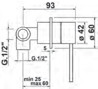
RXD004 • DEVIATORE DOCCIA 2 VIE COMPLETO • COMPLETE 2-WAY SHOWER DIVERTER • INVERSEUR DE DOUCHE 2 VOIES
