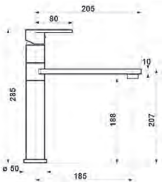
5807 Dandy • MONOCOMANDO LAVELLO • ONE HANDLE SINK MIXER • MITIGEUR ÉVIER
