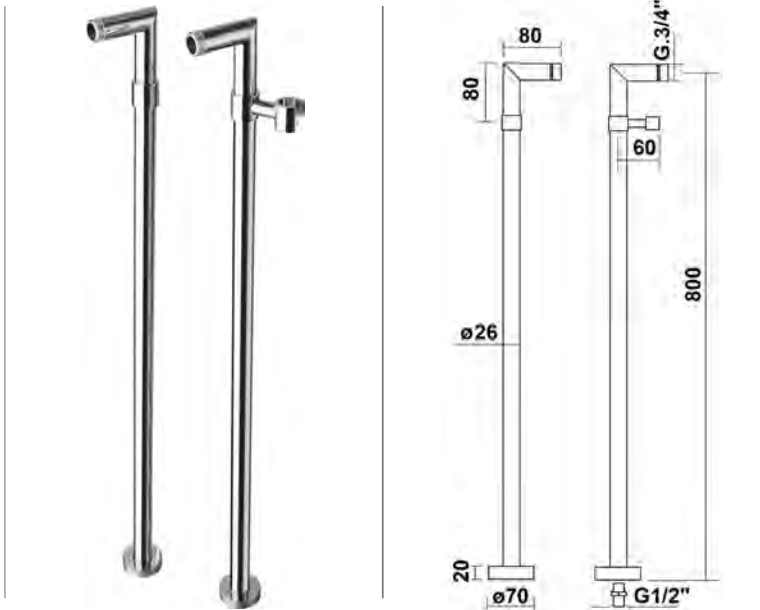
988 • COPPIA COLONNE PER VASCA DA PAVIMENTO • COUPLE OF FLOOR PILLAR LEGS • COUPLE DE COLONNETTES POUR BAIN-DOUCHE
