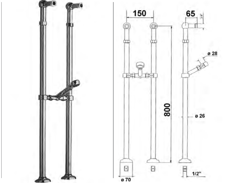
984 • COPPIA COLONNE PER VASCA DA PAVIMENTO • COUPLE OF FLOOR PILLAR LEGS • COUPLE DE COLONNETTES POUR BAIN-DOUCHE
