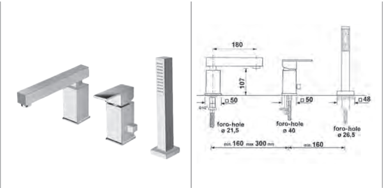
8730 • MONOCOMANDO BORDO VASCA 3 FORI COMPLETO • 3 HOLES DECK MOUNTED BATH SHOWER MIXER WITH SHOWER KIT • MITIGEUR BAIN-DOUCHE 3 TROUS SUR GORGE AVEC ENSEMBLE DE DOUCHE
