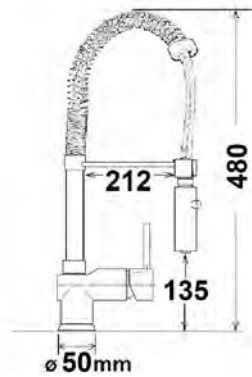
5547 Rhapsody • MONOCOMANDO LAVELLO "PROFESSIONAL" • SINGLE LEVER "PROFESSIONAL" MONO SINK MIXER • MITIGEUR ÉVIER "PROFESSIONAL"
