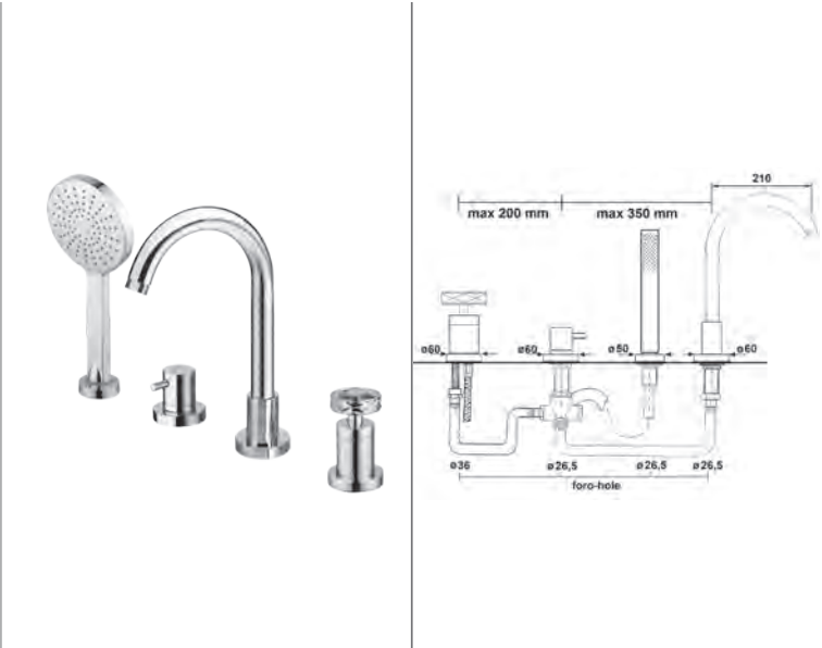
5130RR • MONOCOMANDO BORDO VASCA 4 FORI COMPLETO • 4 HOLES DECK MOUNTED BATH SHOWER MIXER WITH SHOWER KIT • MITIGEUR BAIN-DOUCHE 4 TROUS SUR GORGE AVEC ENSEMBLE DE DOUCHE
